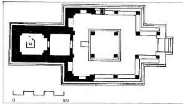
ಕಲ್ಲೇಶ್ವರ ದೇವಾಲಯದ ತಲವಿನ್ಯಾಸ
