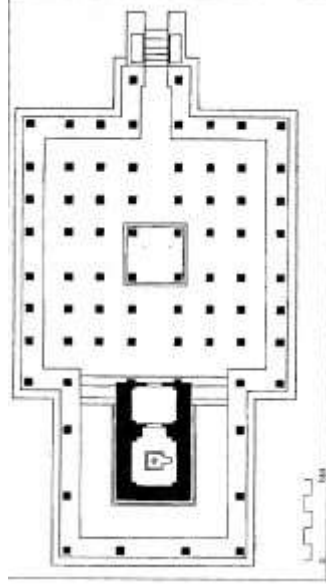
ಹಿಂಡುಲಿ ಸಂಗಮೇಶ್ವರ ದೇವಾಲಯದ ತಲವಿನ್ಯಾಸ
