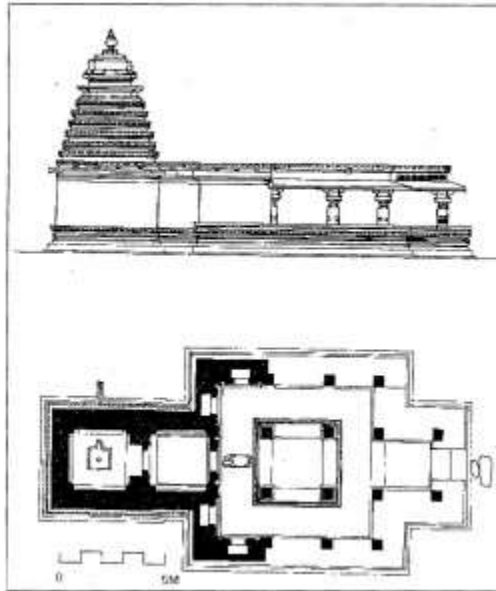
ಉಜಾಳೇಶ್ವರ ದೇವಾಲಯದ ತಲವಿನ್ಯಾಸ
